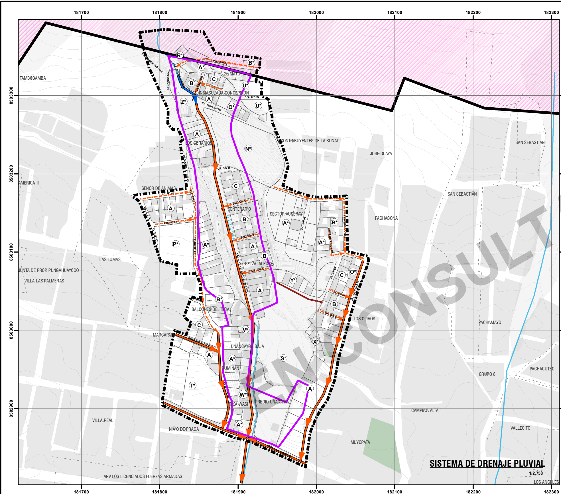
SUMIDEROS COLECTORES UBICADOS CADA 100 m. EN CALLE JUAN VELASCO ALVARADO
